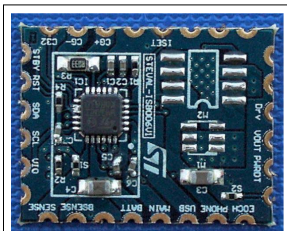
STEVAL-ISB006V1
